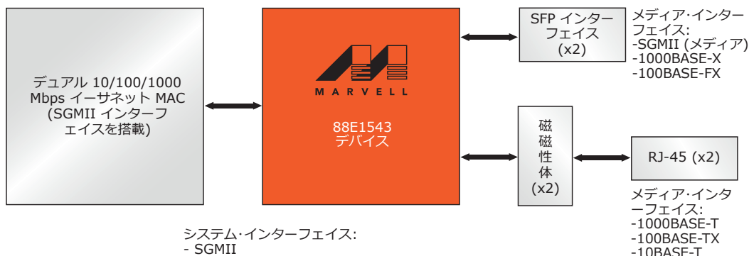
図 2: デュアルポート SGMII (システム)~メタル/SGMI/ファイバー (自動メディア検知)
